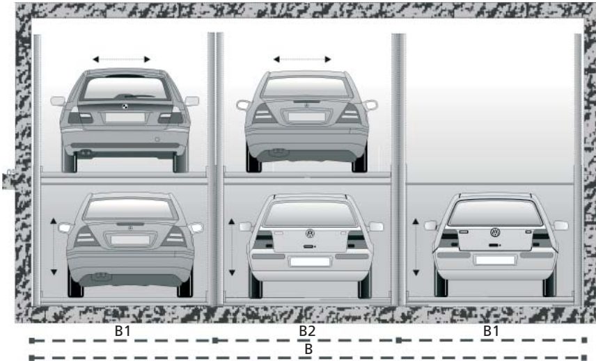
Breitenmaße, Abb. 3 Segmente für 5 Stellplätze
